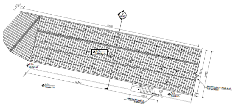
د دوېم پور د بام نڅېنه (نقشه)
