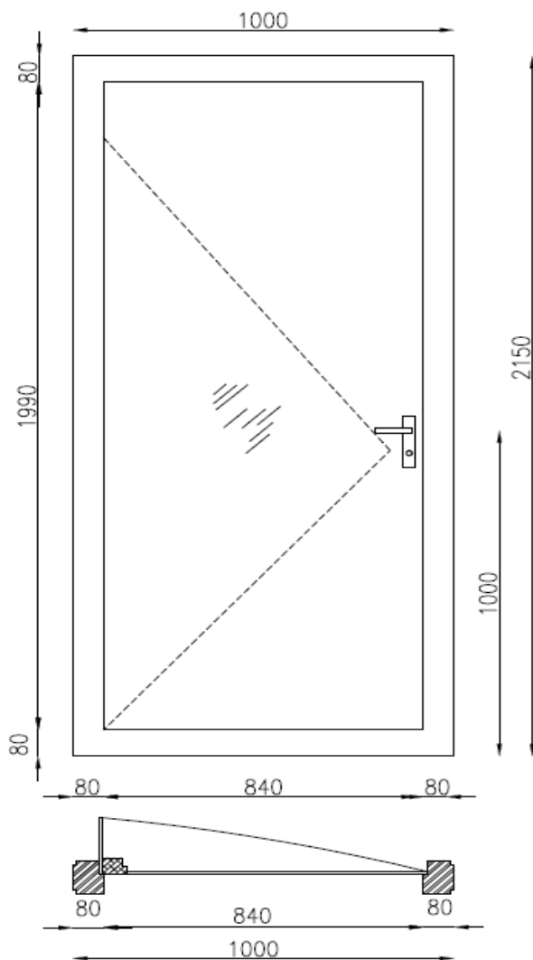
د ودانۍ د یوې دروازې انځور
