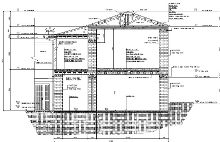
د ودانۍ پریک ( قطع یا برش) نڅښه (نقشه)
