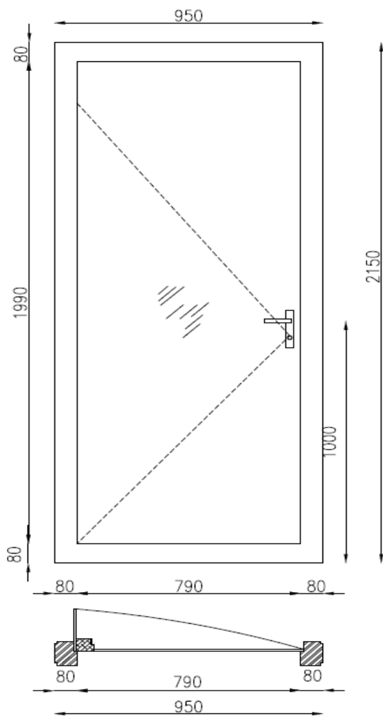
د ودانۍ د یوې دروازې انځور
