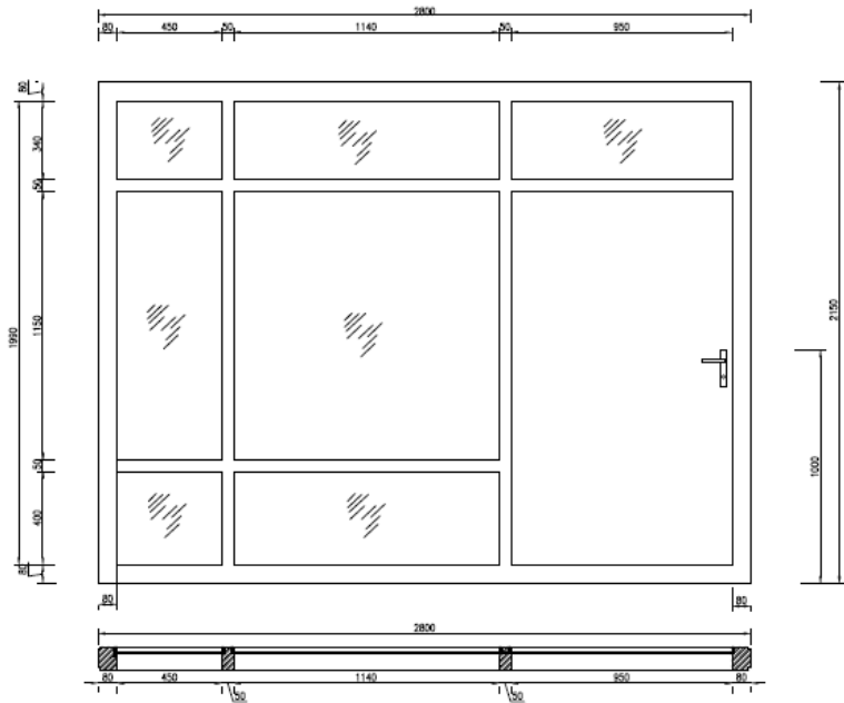
د ودانۍ لمړي پور دروازې / کرکی انځور
