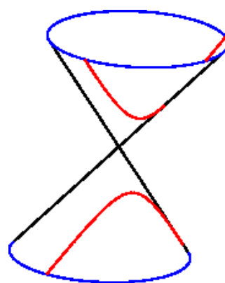
Hyperbolic: های پارابول \beta < \alpha/2
