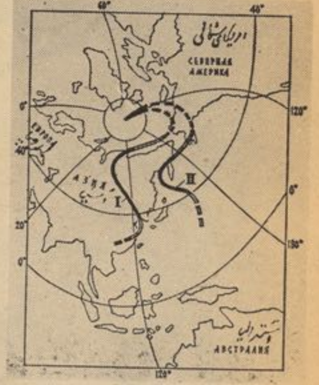
منحنی (قطب های سرگردان) که نظریه معلومات پالئو مغناطیسق برای اروپا و امریکای شمالی «۱» بدست آمده است اگر هر دو براعظم باهم وصل شوند ، منحنی ها باهم منطبق خواهند گردید .
