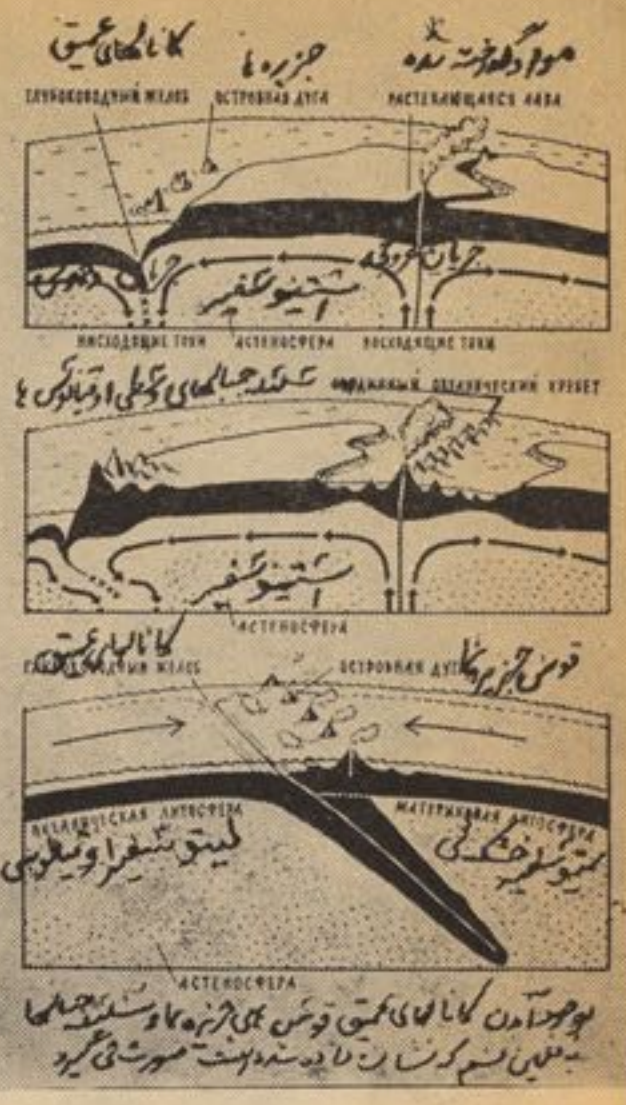
وجود آمدن کانا لهای عمیق قوس های جزیره نما و سلسله جانی به همین قسم که نشان داده شده است صورت میگرد .
