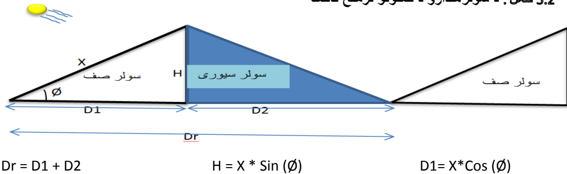
5.2 شکل : د سولر هندارو د صفونو ترمنځ فاصله
