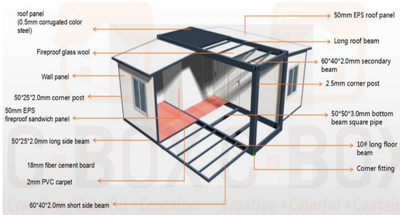
د جلا کېدو وړ کانتینر تشریح انځور
