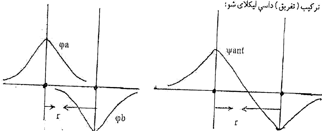
شکل (2 - 31): په H_2^+ ايون کې ضد اړتيايي ماليکولي اړتال \psi_{ant} جوړيدل. r - د هستو تر منځ فاصله
