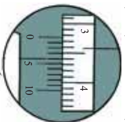
(9-1) شکل، د ورنیر کالیبر د خط کش درجې د ویلو سمه طریقه
