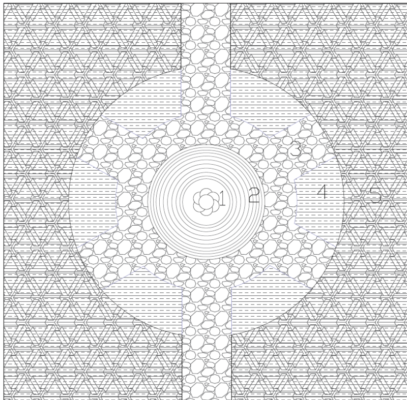
د وچ بن یوې کوچنۍ بېلگې پلان
