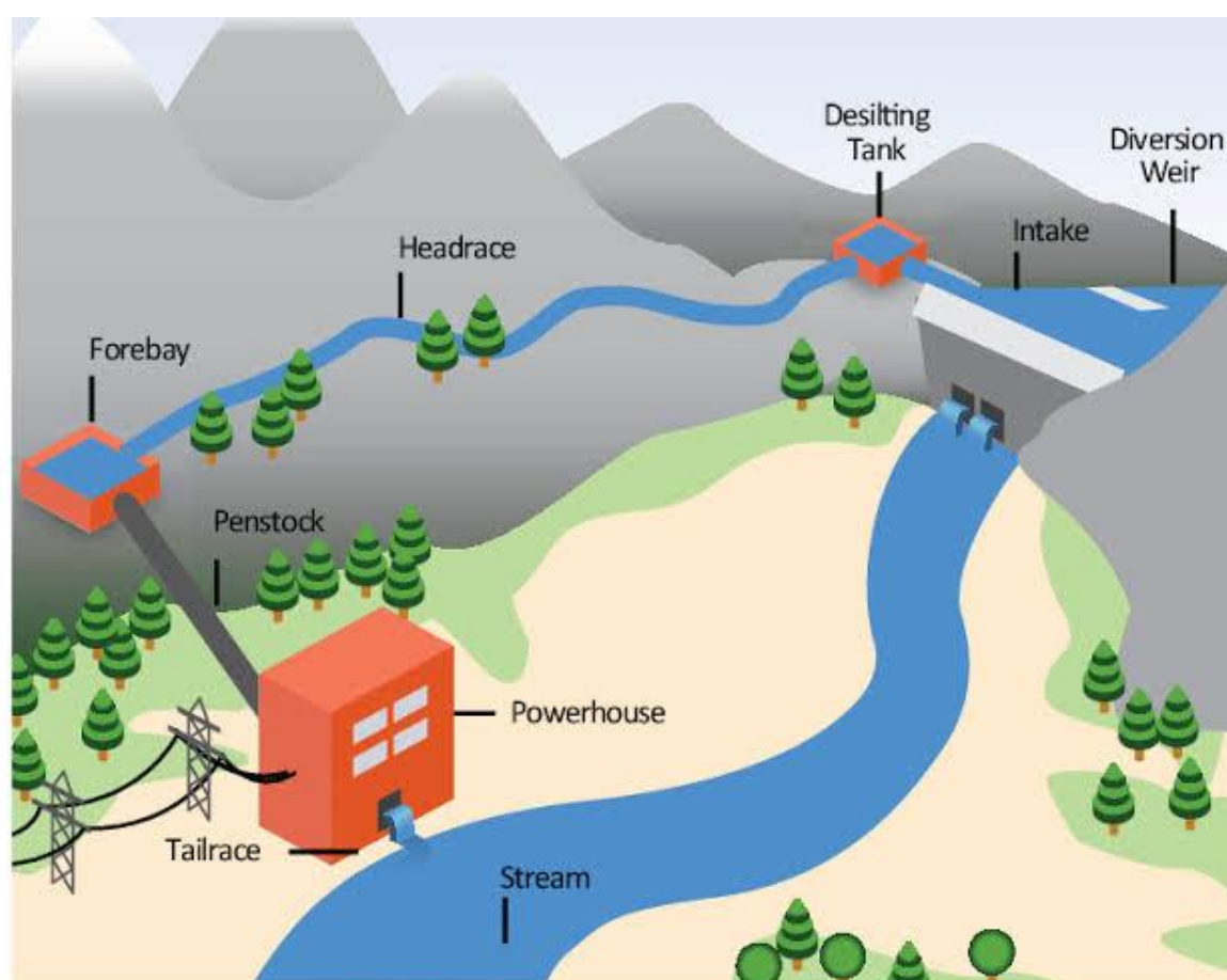
2.2 شکل: د اوبو د کوچنۍ برېښنا بند مختلف ساختمانونه
