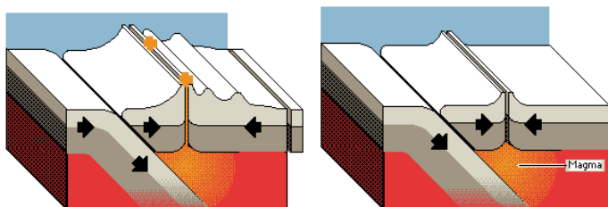
پروسه حرکت متداوم قشر زمین (Plate Tectonic)
