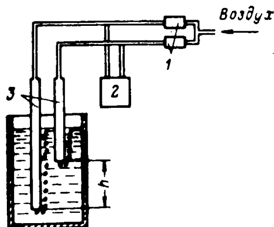
شیمای کثافت سنج هایدروستاتیکی با هوا دهی
