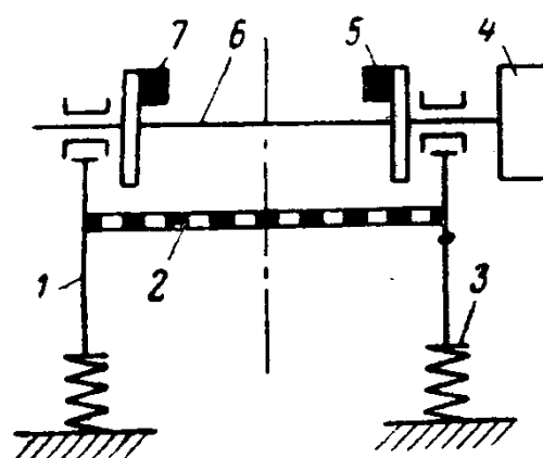
شیمای غربال اهتزاز
