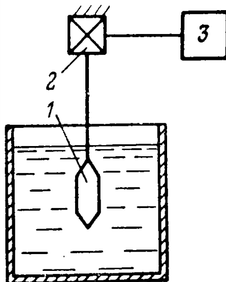
شیمیای کثافت سنج با شناور غرقى
