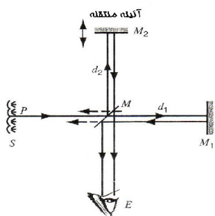
شکل ۳ - ۲۰ : تداخل سنج مایکل سن نشان
