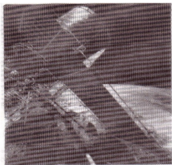
شکل ۲ - ۳۱ :- تلسکوپ فضائی هوبل.
