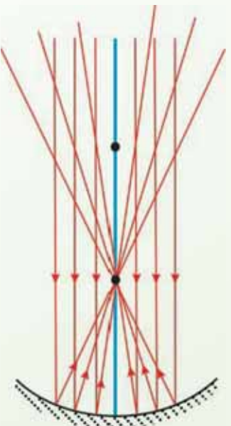
د (3-19) شکل هغه وړانگې چې له اصلي محور سره موازي دي په مقعره هنداره باندې واردېږي، له انعکاس څخه وروسته له اصلي محراق څخه تېرېږي.
