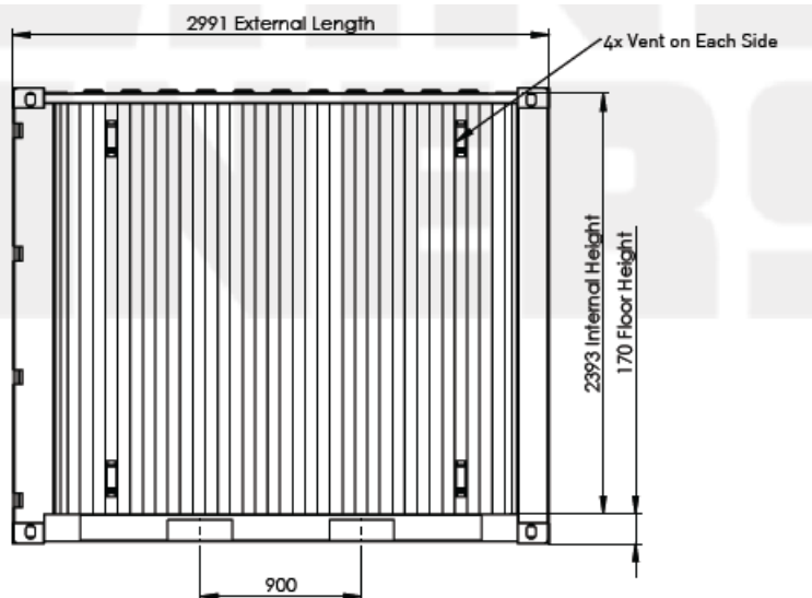
د ۱۰ فته مینی کانتینر اړخ لید
