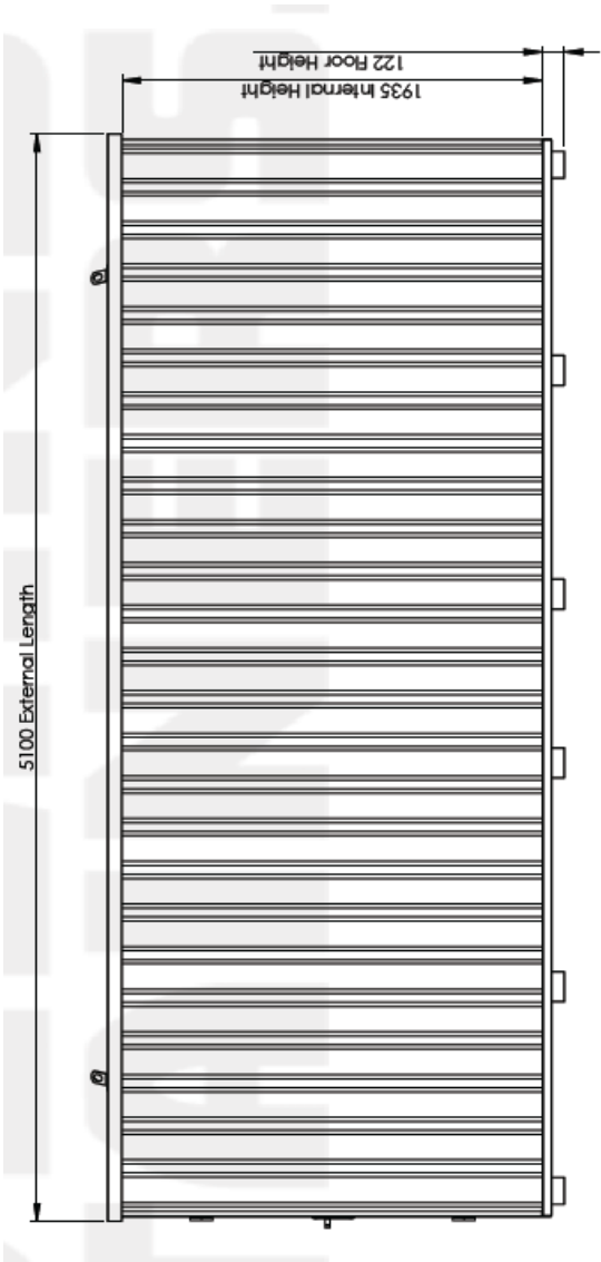
د فلت پک کانتینر ۵ په ۲ مترو کې، اوږد اړخ لید
