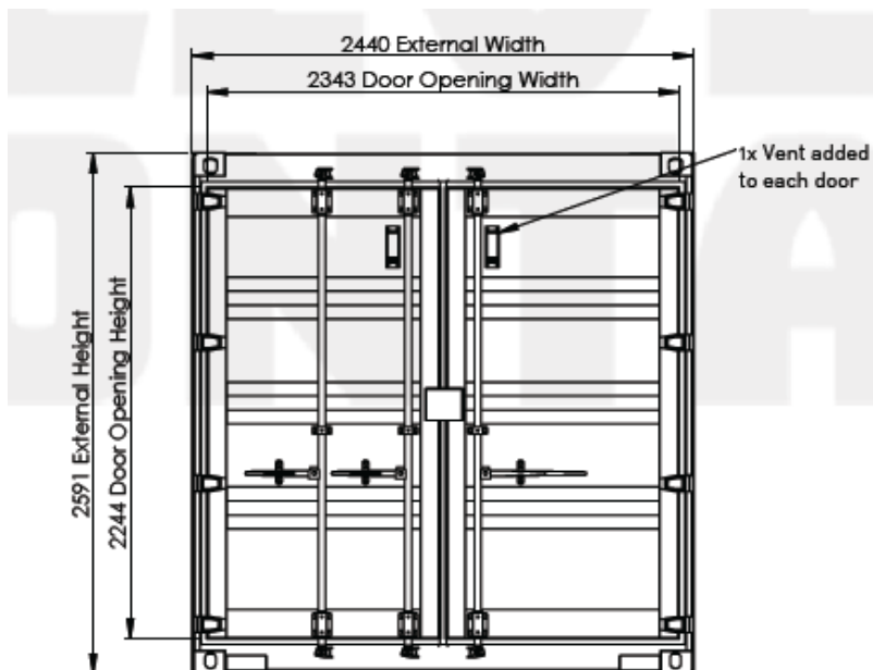
د ۱۰ فته ډیپوکانټینر دروازې لید
