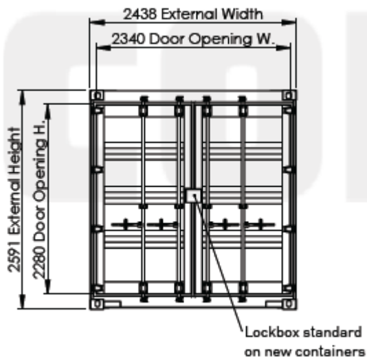
د ۴۵ فته ستنډرډ کانتینر دروازي لید
