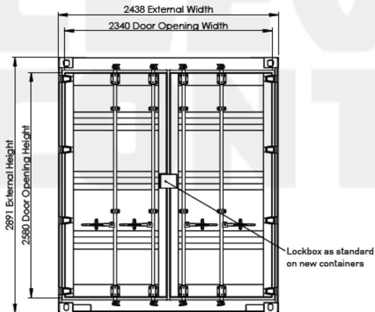
د ۲۰ فته اوجت کانتینر دروازی لید
