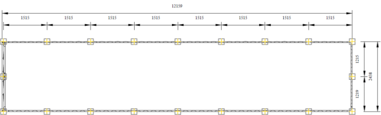
د ۴۰ فوټ کانتینر له پاره د کانکریت بلاک پلان ۲۰۰ x ۲۰۰ ملی متر ، نښه ۱:۳
