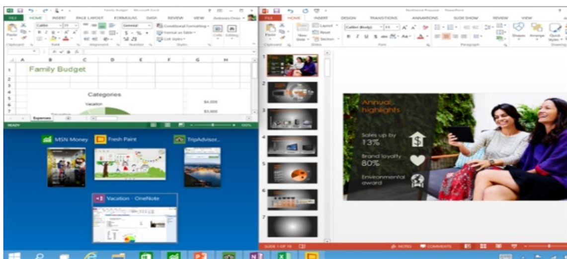
۸.۶ Snap Assist
