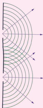
شکل، (2-21) د نوري وړانگو تداخل بڼه
