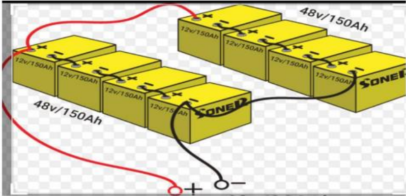
۲۲-۳ انځور: د بطریو مسلسله تړنه
