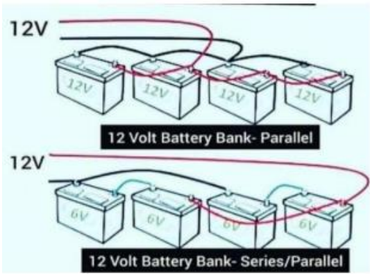
۲۳-۳ انځور: د بطریو مسلسل او موازي تړنه
