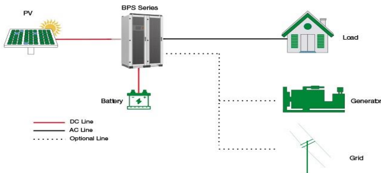
۲-۴ شکل: د هایبرېډ اېنورټر د اتصال انځوریزه شیمه
