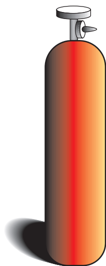
(۱-۹) شکل: د کاربن ډای اکسایډ ګاز
