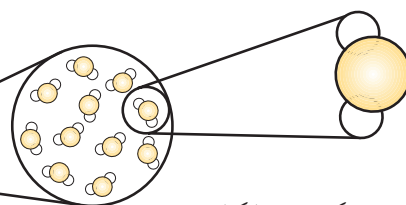
(۱-۸) شکل: د اوبو مالیکولونه
