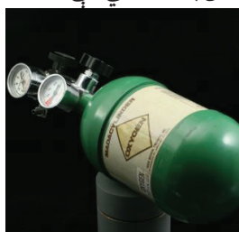
(۷-۴) شکل: په کپسول کې څیرمه شوي اکسیجن
