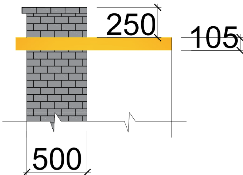
دیتایل ۱ در قطع یا تراش بدون در نظر داشت خشت کاری
